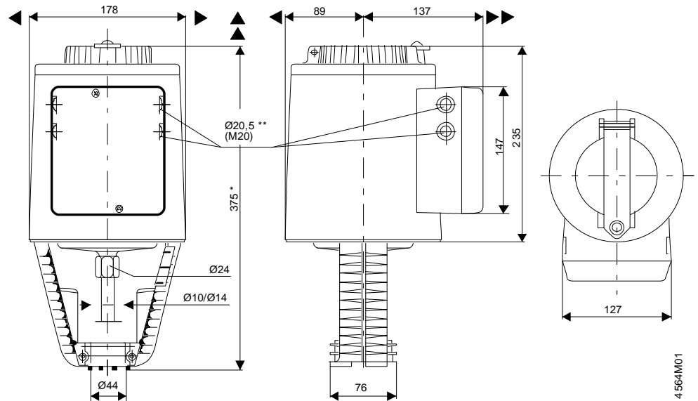
尺寸 (mm)
